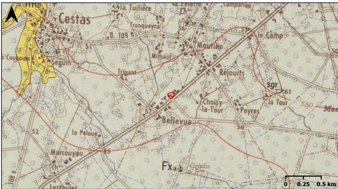
Extrait de la carte géologique de Pessac
